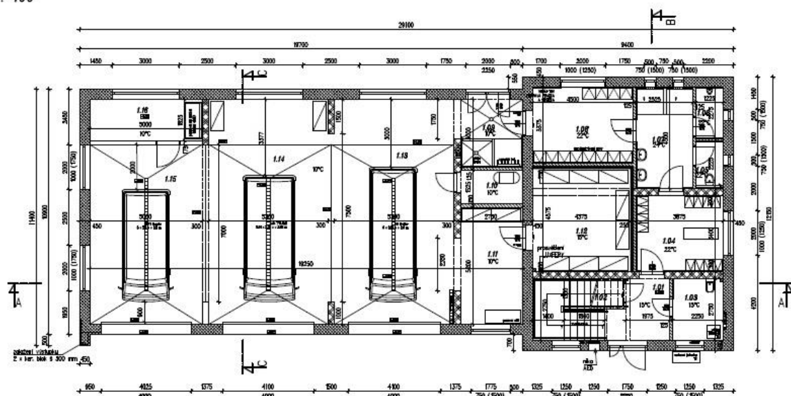
Půdorys přízemí M = 1 : 100
